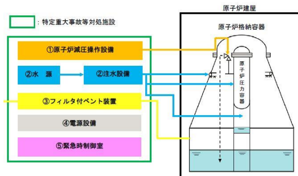
特定重大事故等対処施設の概要図(原電の申請文書より)
